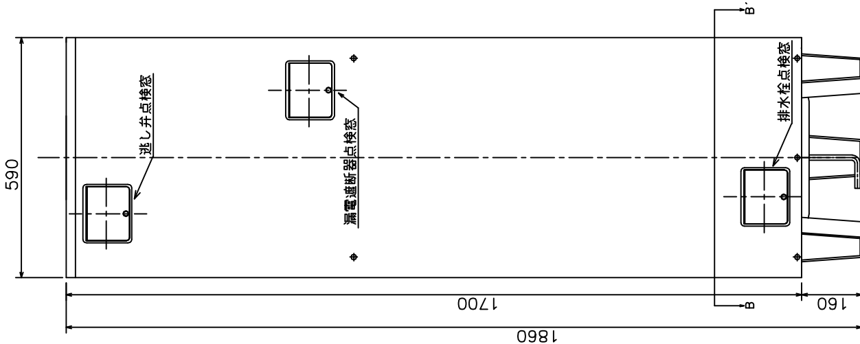
正面図
