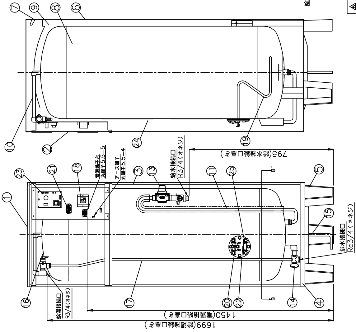
正面図
