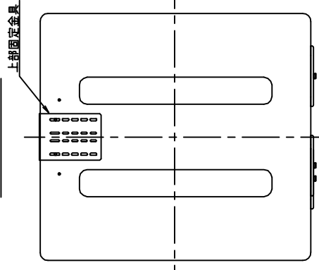
上面図
