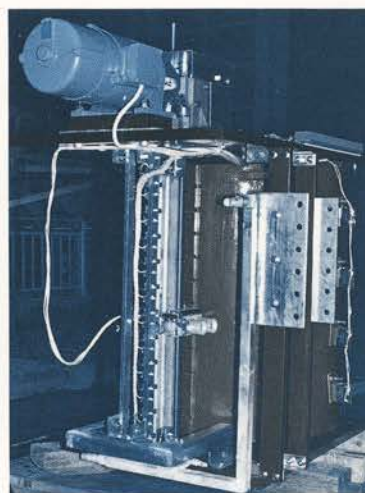
水冷空心可変容量リアクトル (Water Cooled Air Core Variable Capacity Reactor) 2400kVA
