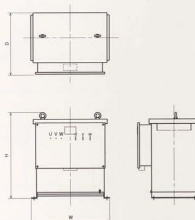
DWG ④
