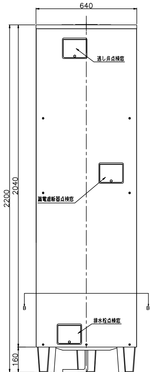
正面図
