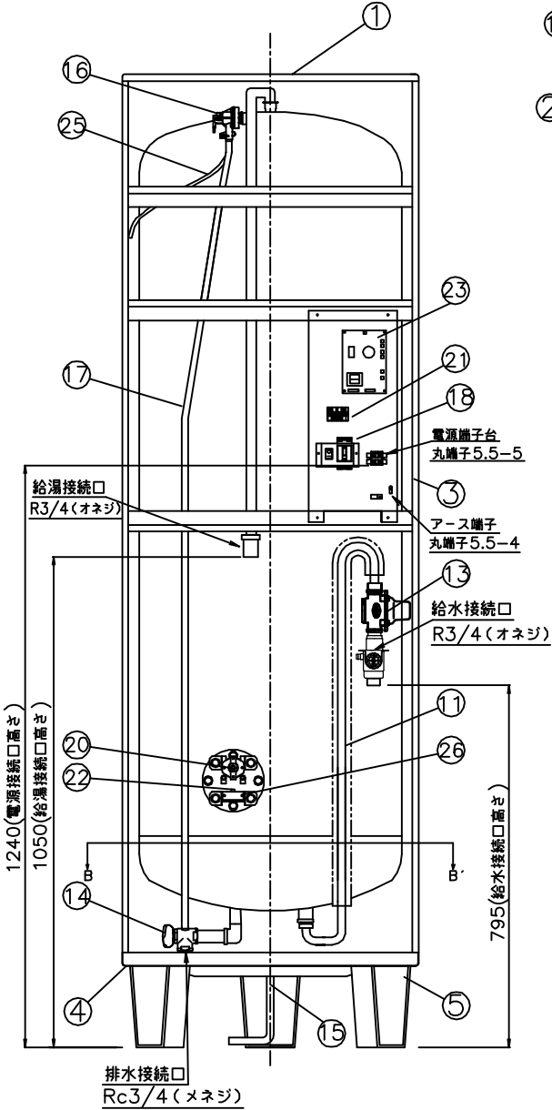
正面図
