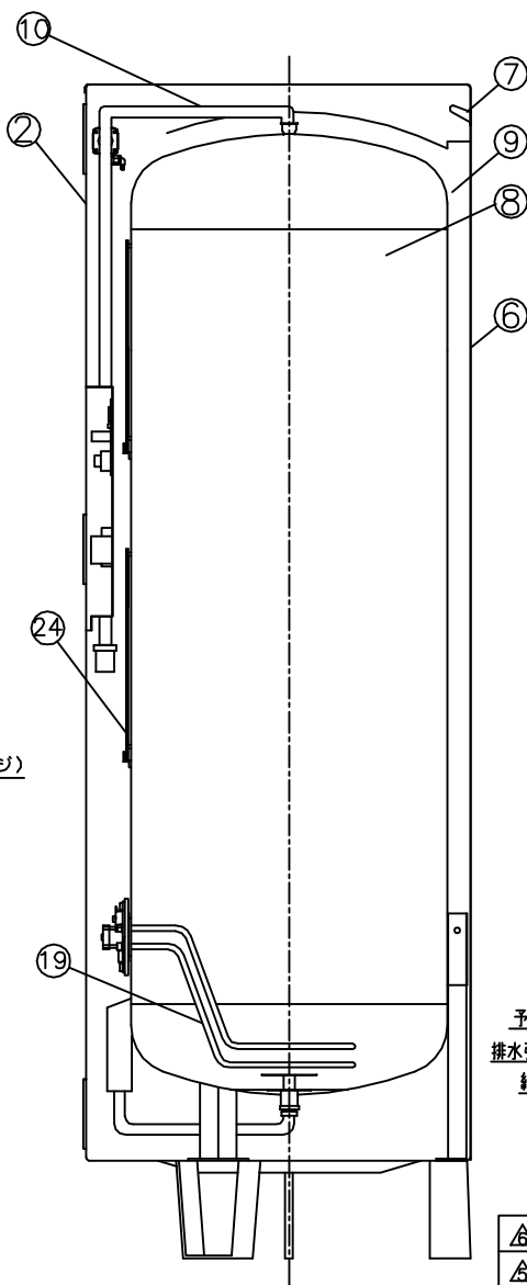
側面図
