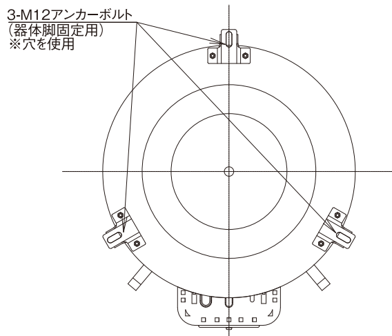
アンカーボルト位置(上面透視図)
