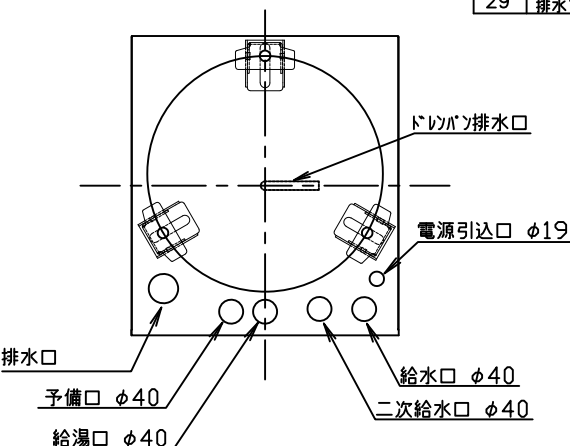
B-B'断面図(上から見た図)
