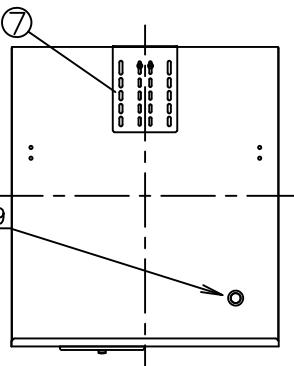
上面図
