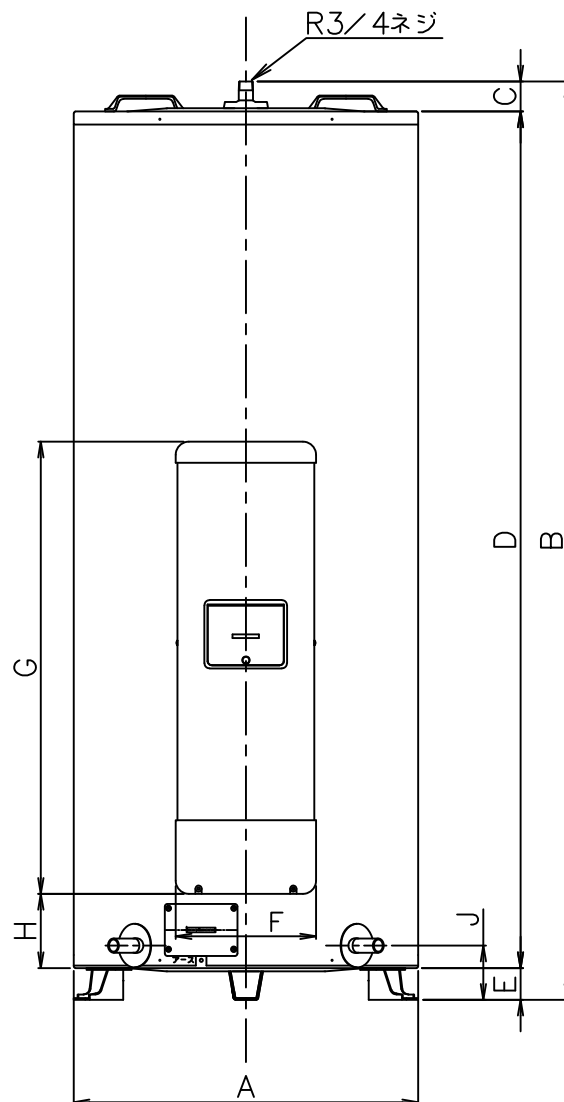
正面図
