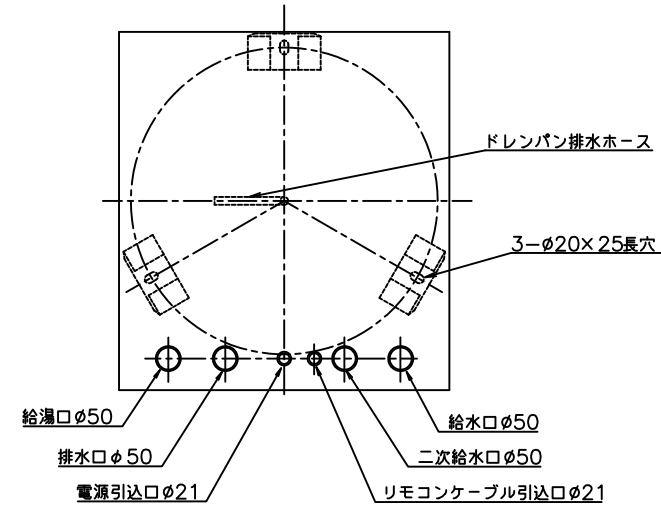
B-B' 断面図 (上から見た図)
