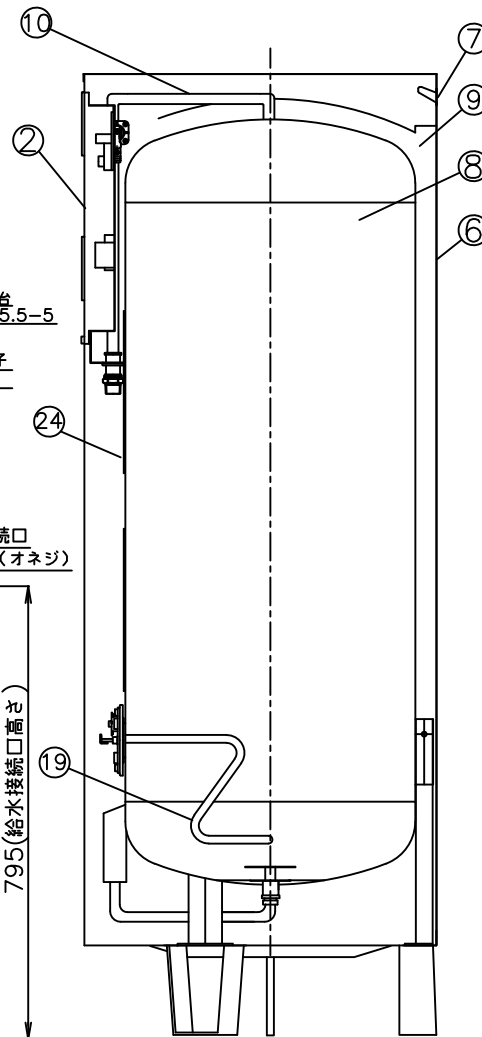
側 面 図
