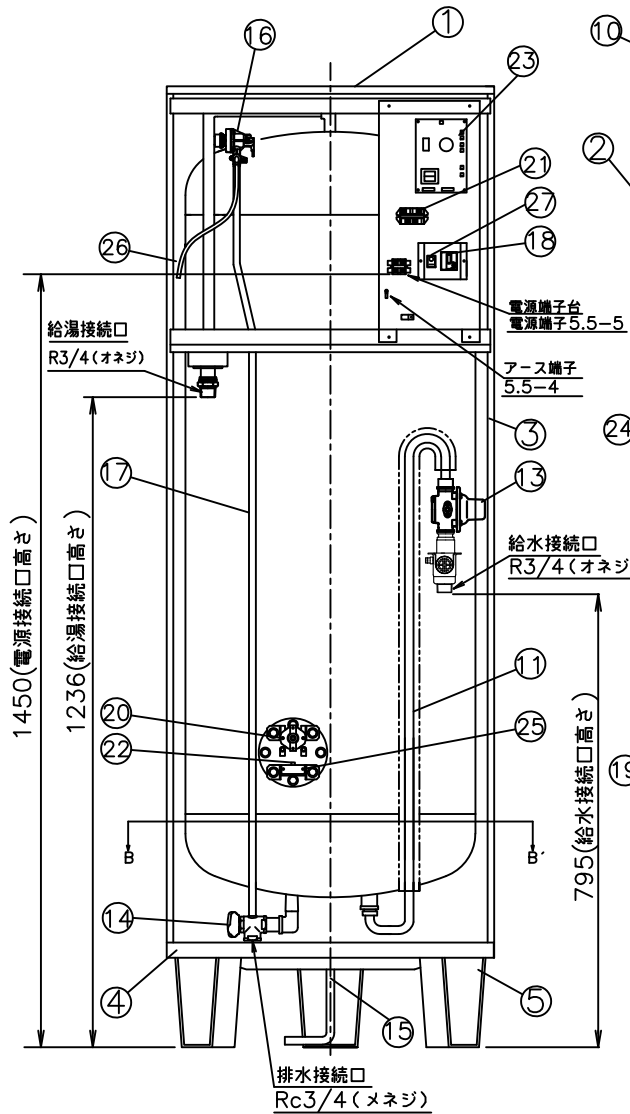
正面図
