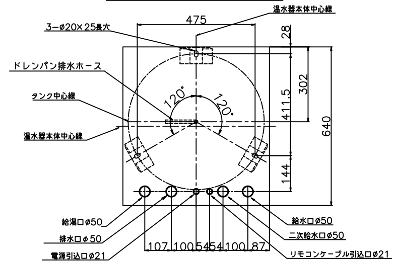
B-B' 断面図(上から見た図)
