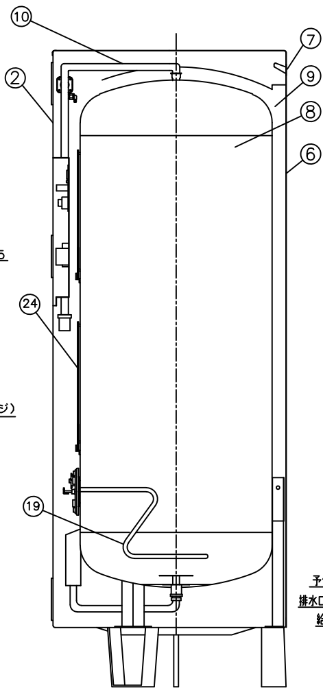
側面図
