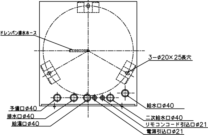
B-B' 断面図 (上から見た図)
