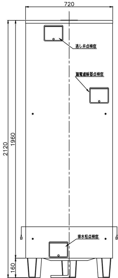
正面図
