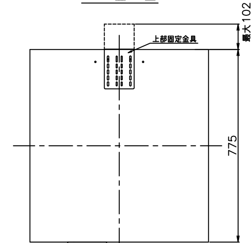
B-B'断面図 (上から見た図)
