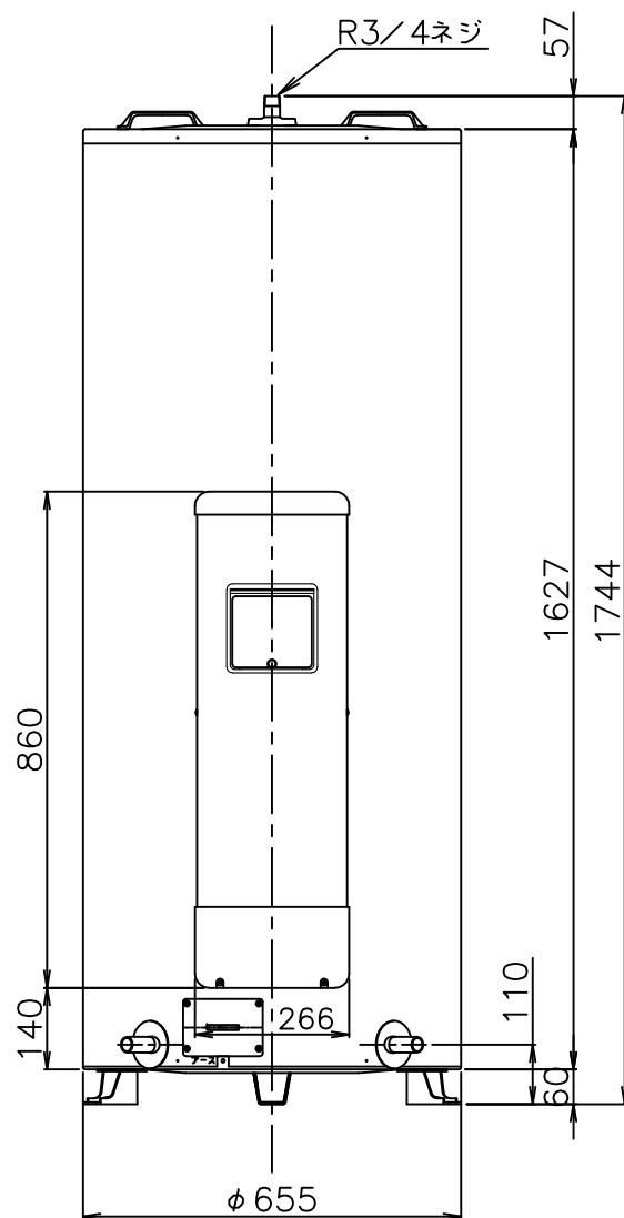
正面図
