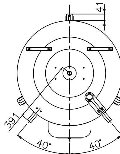
底面図
